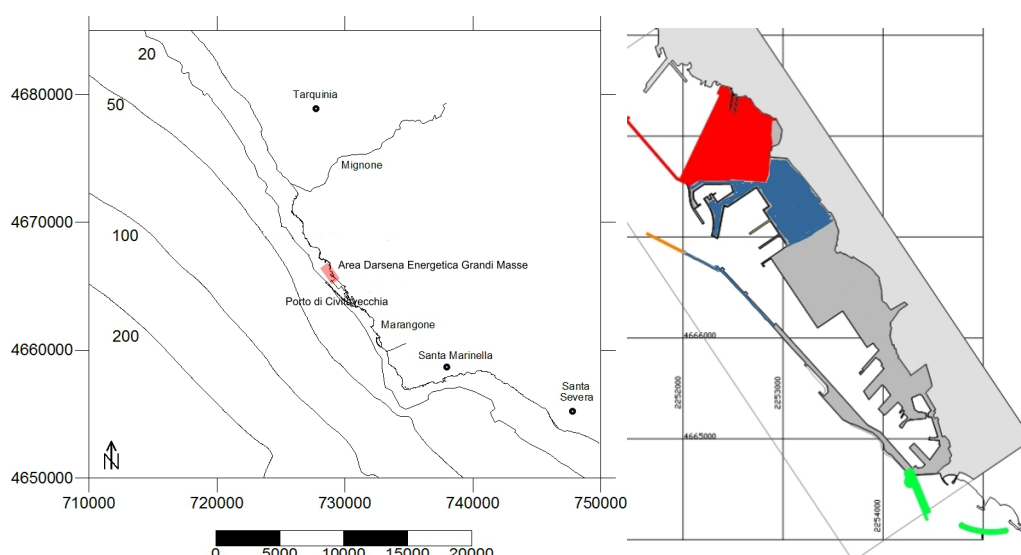
Fig. 2 Area costiera di Civitavecchia (sinistra) e planimetria delle opere nel Porto di Civitavecchia. In azzurro l'area di intervento per il I Lotto Funzionale Opere Strategiche
