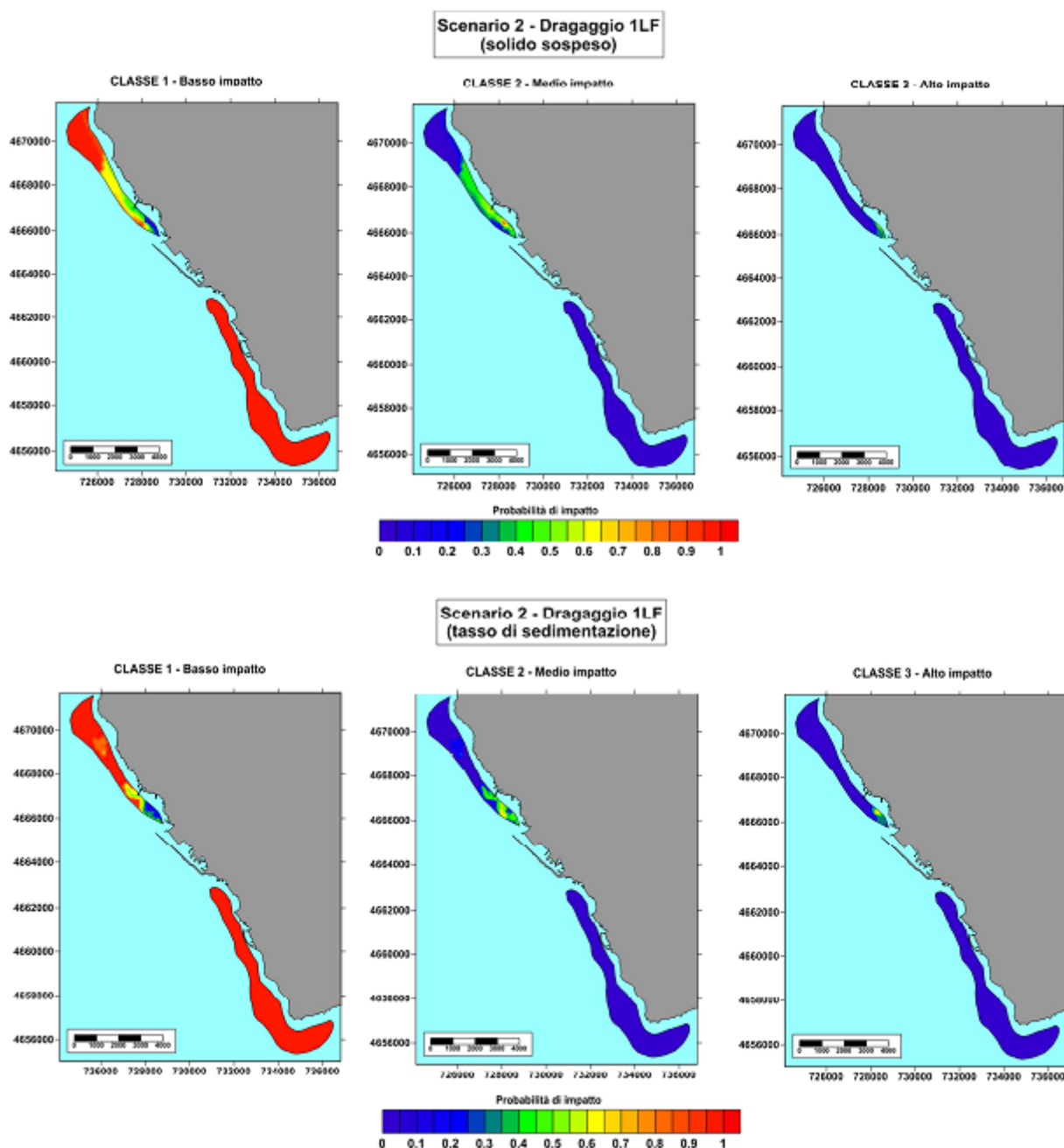
Fig. 9 Mappe dell'indice D3I per bassa, media e alta probabilità d'impatto dovuti alle operazioni di dragaggio per le opere del 1LF. In alto gli impatti generati dal sedimento in sospensione, in basso quelli dovuti al tasso di sedimentazione.
