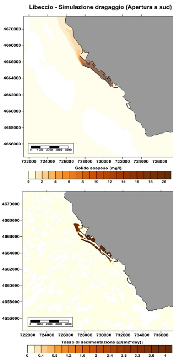
Fig. 12 distribuzione del solido in sospensione (in alto) e del tasso di sedimentazione (in basso) dovuto alle operazioni di dragaggio per le opere del 2LF (Apertura a sud) (Libeccio).
