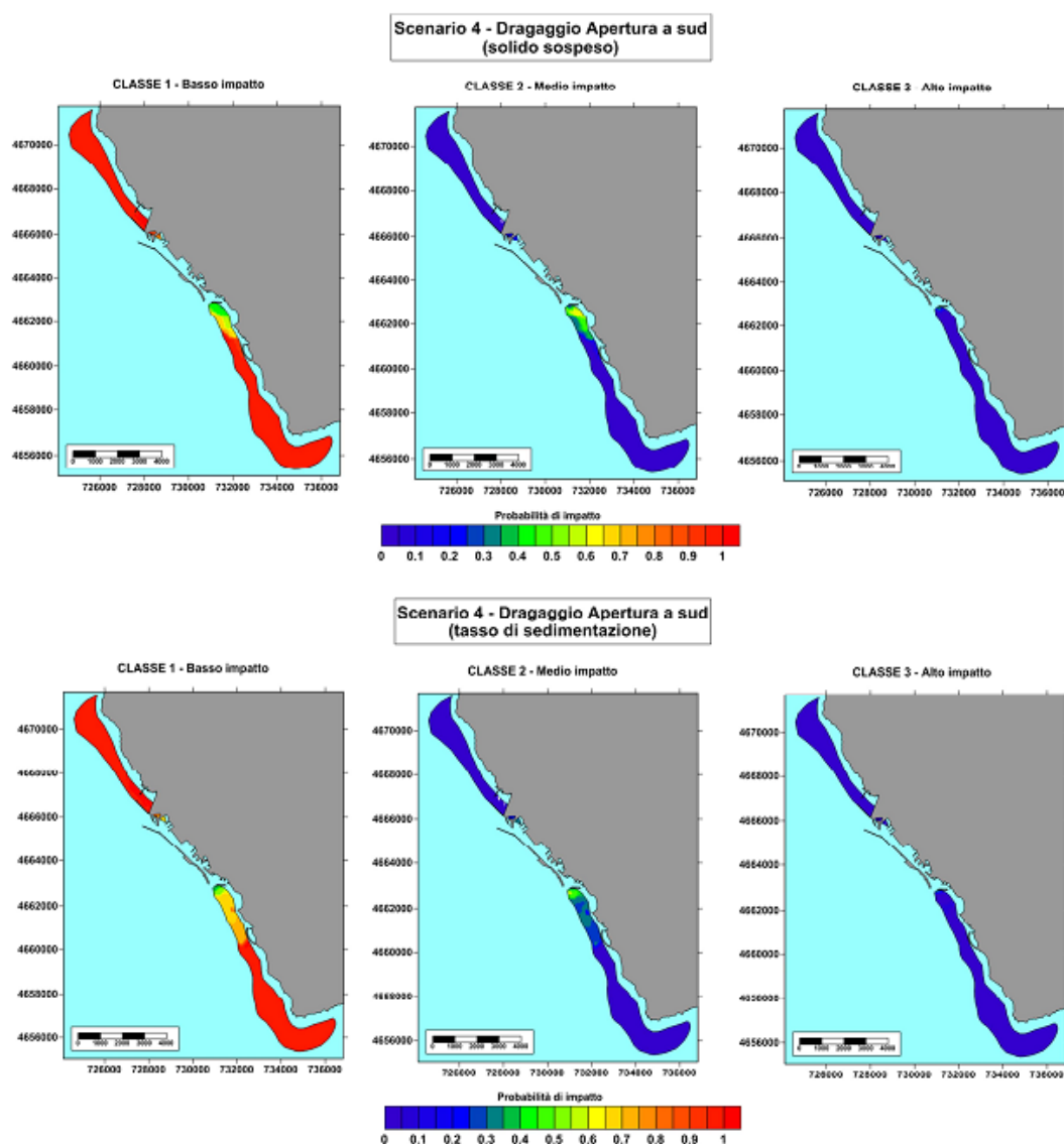
Fig. 13 Mappe dell'indice D31 per bassa, media e alta probabilità d'impatto dovuti alle operazioni di dragaggio per le opere del 2LF (Apertura a sud). In alto gli impatti generati dal sedimento in sospensione, in basso quelli dovuti al tasso di sedimentazione.
