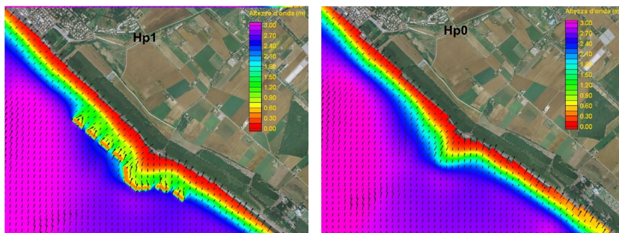
Fig. 15 Effetto di una barriera soffolta sulle mareggiate incidenti lungo la linea di costa.
