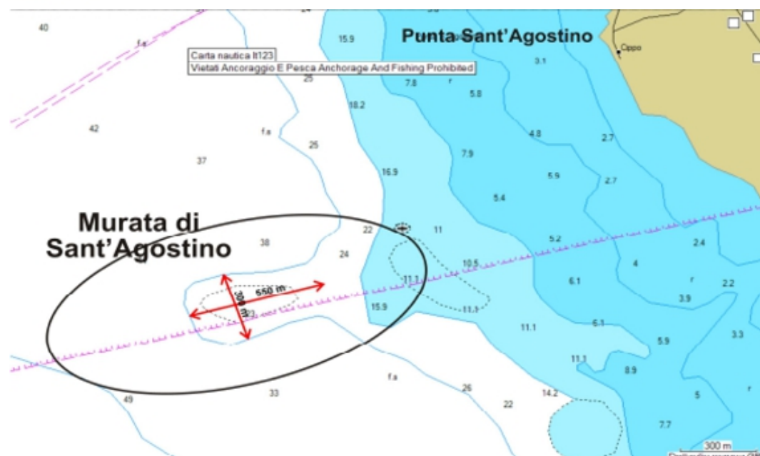
Fig. 36 Struttura e dimensioni della Murata di Sant'Agostino.
