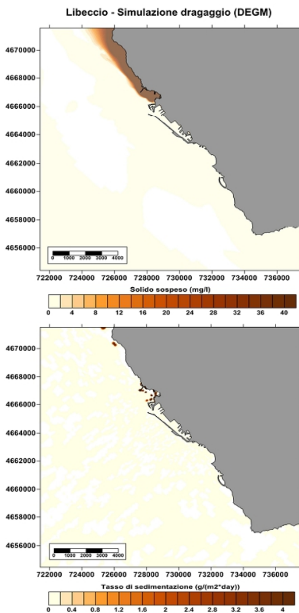
Fig. 10 distribuzione del solido in sospensione (in alto) e del tasso di sedimentazione (in basso) dovuto alle operazioni di dragaggio per la DEGM (Libeccio).
