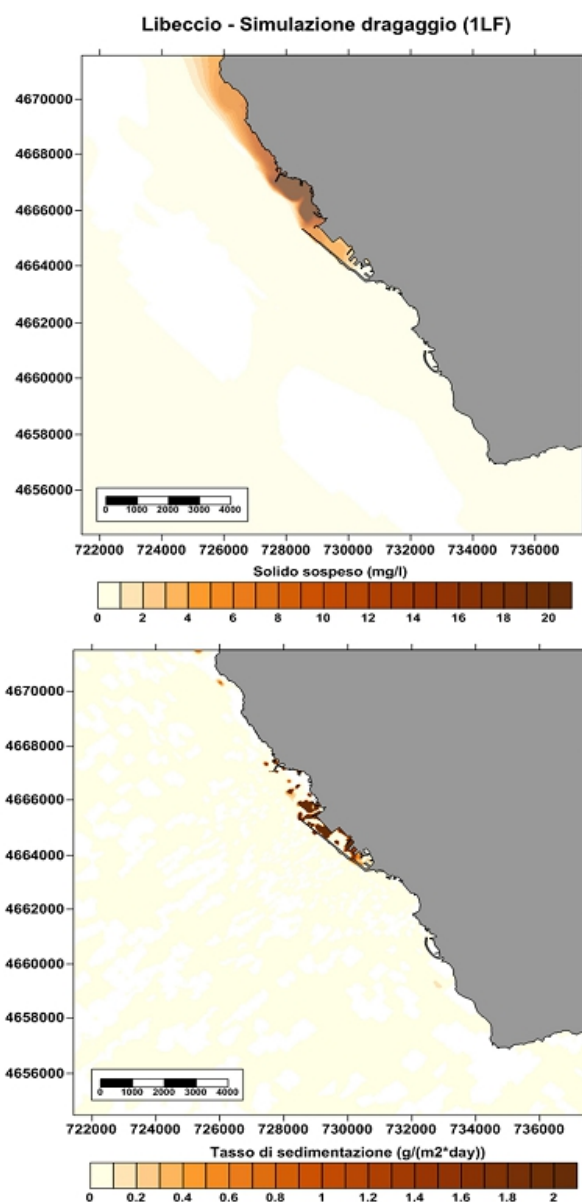
Fig.8 distribuzione del solido in sospensione (in alto) e del tasso di sedimentazione (in basso) dovuto alle operazioni di dragaggio per le opere del 1LF (Libeccio)
