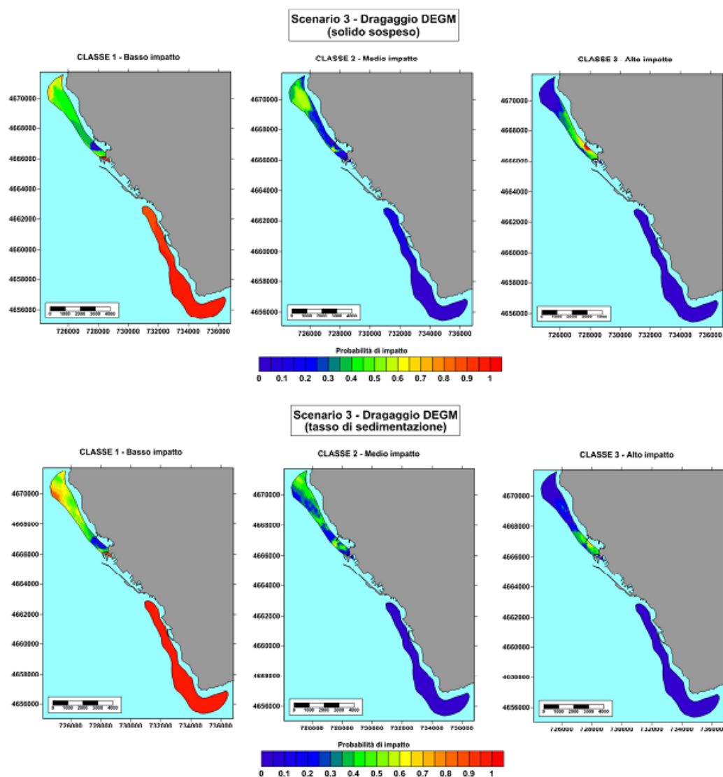
Fig. 11 Mappe dell'indice D3I per bassa, media e alta probabilità d'impatto dovuti alle operazioni di dragaggio per le opere della DEGM. In alto gli impatti generati dal sedimento in sospensione, in basso quelli dovuti al tasso di sedimentazione.
