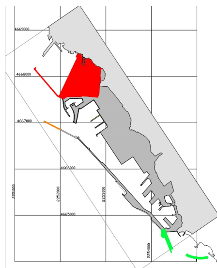
Fig. 4 Area costiera di Civitavecchia (sinistra) e planimetria delle opere nel Porto di Civitavecchia. In verde l'area di intervento per il II Lotto Funzionale O.S
